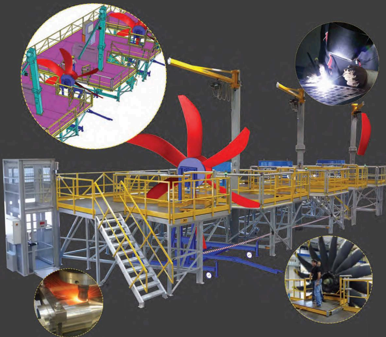
Projet Plate-forme d'assemblage
